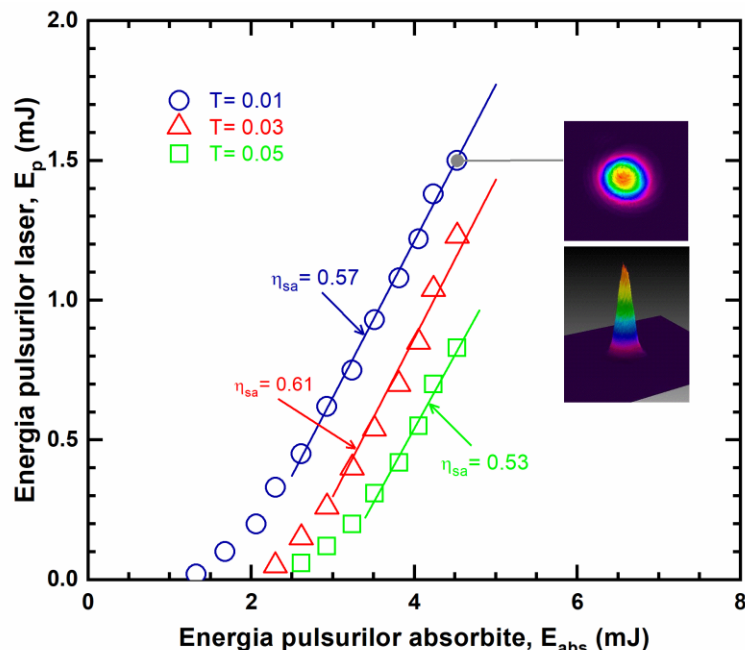
Figura 10. Energia pulsurilor laser generate de cristalul 4 at.% Yb:LYSB în funcție de energia pulsului de pompaj absorbită ( E_{abs} ). T reprezintă transmisia oglinzii de extracție OCM.
