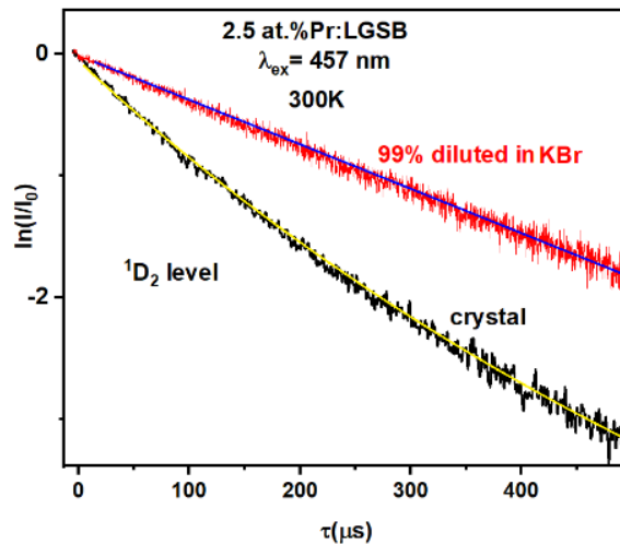
Figura 16. Cinetica emisiei la 300K a nivelului {}^1\text{D}_2 al ionilor \text{Pr}^{3+} în cristalul 2.5 at.% Pr:LGSB. [20]
